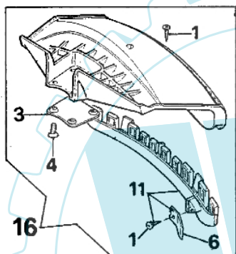
mod. 722S - 726S - 726D 726T - SPARTA 26
