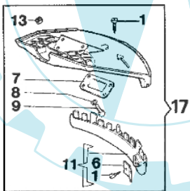
mod. 722S - 726S - 726D 726T - SPARTA 26
