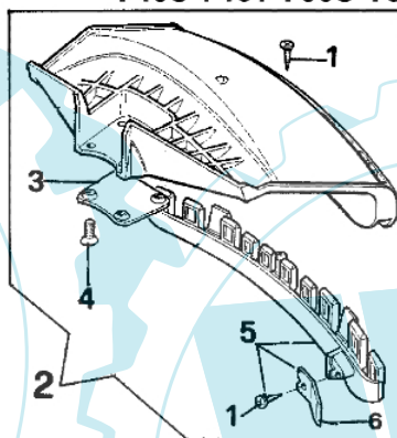
mod. TR 60 E - SPARTA 26 TR
