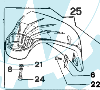
mod. 720 - TR 100 E
